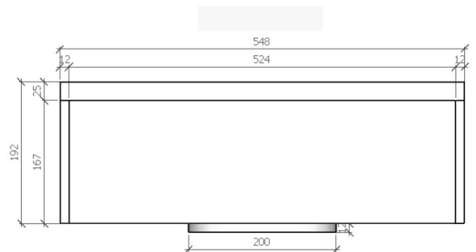
VISTA TRASEIRA
