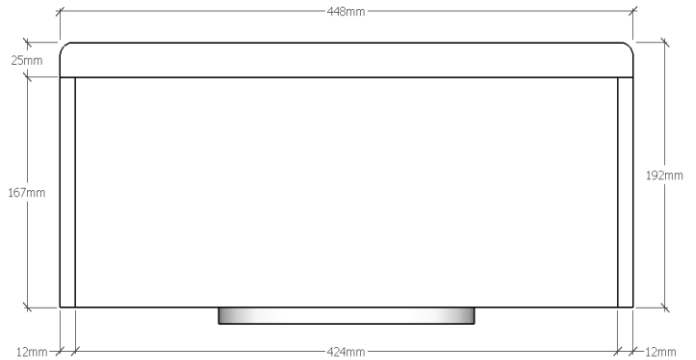
VISTA TRASEIRA
