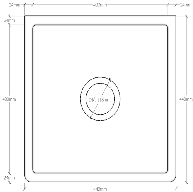
VISTA SUPERIOR
