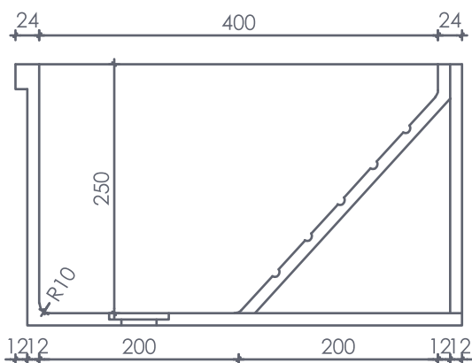
CORTE
