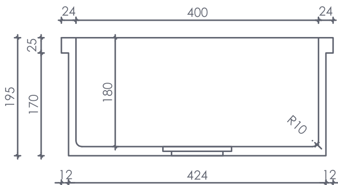
CORTE TRANSVERSAL
