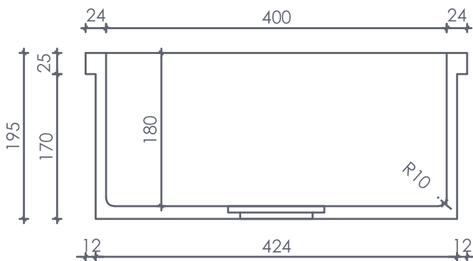
CORTE TRANSVERSAL
