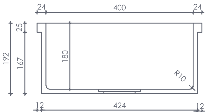
CORTE TRANSVERSAL
