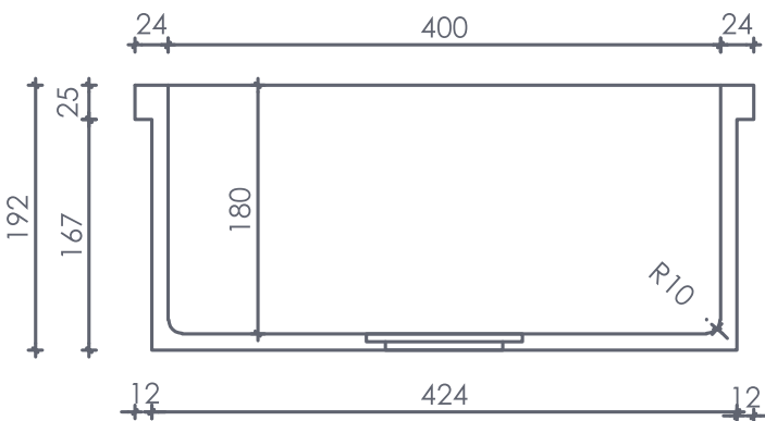
CORTE TRANSVERSAL
